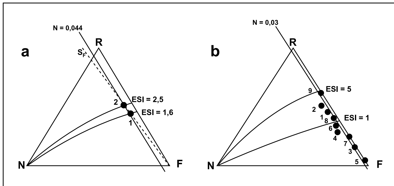
Figura 7: Diagramas emergéticos ternários representando (a) produção de soja com fertilizantes químicos (1) e com inoculação de Bradhyrizobium japonicum (2) e (b) milho na Itália (3), milho na Toscana (4), girassol na Itália (5), girassol na Toscana (6), cereais na Toscana (7), forragem na Itália (8) e forragem na Toscana (9).
