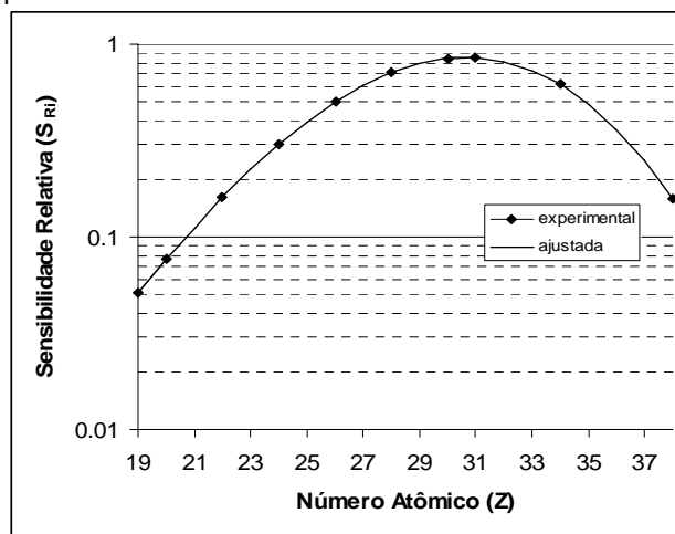
Fig. 3 – Curva da sensibilidade relativa ( S_{Ri} ) para série K utilizando SR-TXRF.
