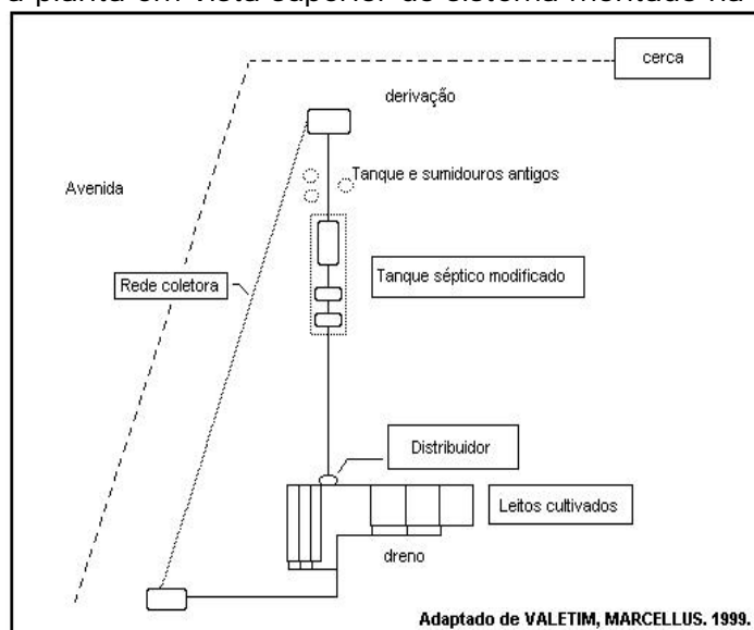
Fig. 1 – Planta superior do sistema de tratamento de esgoto doméstico da FEAGRI.
